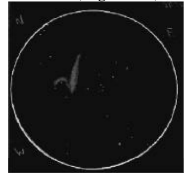
M17 (Sagittarius)
