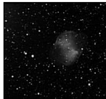
M27 (Vulpecula)
