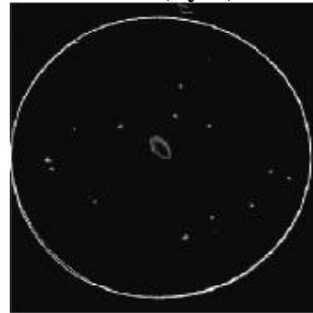
M57 (Lyra)
