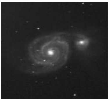
M51 (Canes Venatici)
